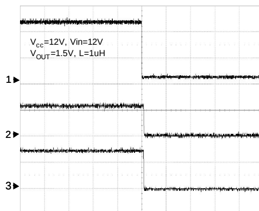
Shutdown (V EN =V GND )
